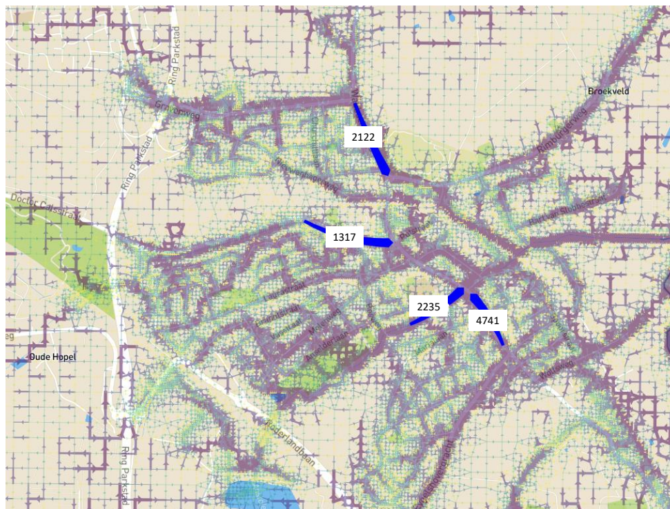
Figuur 22. Totale afstroomvolumes (eerste twee uur van de simulatie) langs de belangrijkste routes bij het T=100 -scenario
