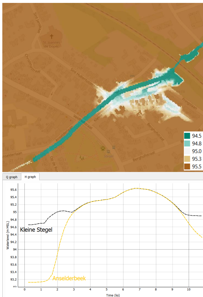
Figuur 24. Waterstandsverloop op de Kleine Stegel en de Anselderbeek bij neerslagsscenario Regenradar 29 juni 2021
