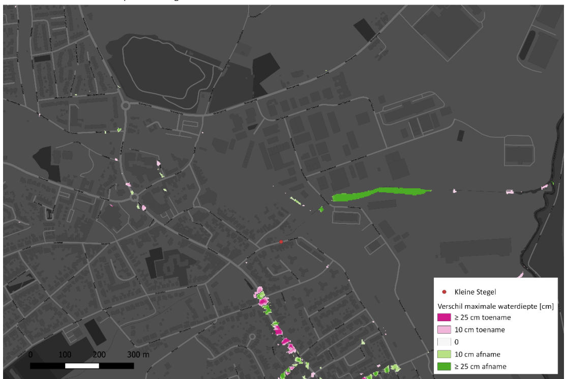
Vershil maximale waterdiepte: maatregel D t.o.v. verwacht T100
