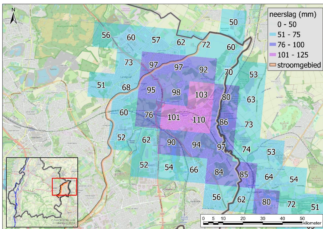
Figuur 8 Totaal neerslagvolume van 29 juni 10:00 tot 30 juni 10:00, totaal overzicht (boven) en ingezoomd op Eigelshoven (onder)
