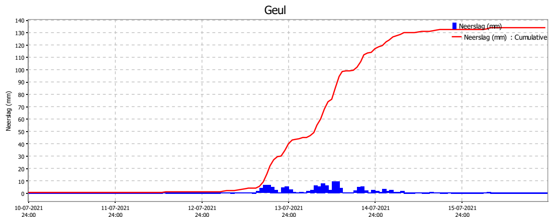
Figuur 8 Neerslagverloop voor het stroomgebied van de Geul (gebiedsgemiddelde)
