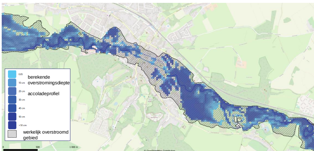
Figuur 30 Overstroomde gebieden in en nabij Valkenburg na realisatie van het accoladeprofiel in het centrum van Valkenburg tussen Walramstuw en Odapark
