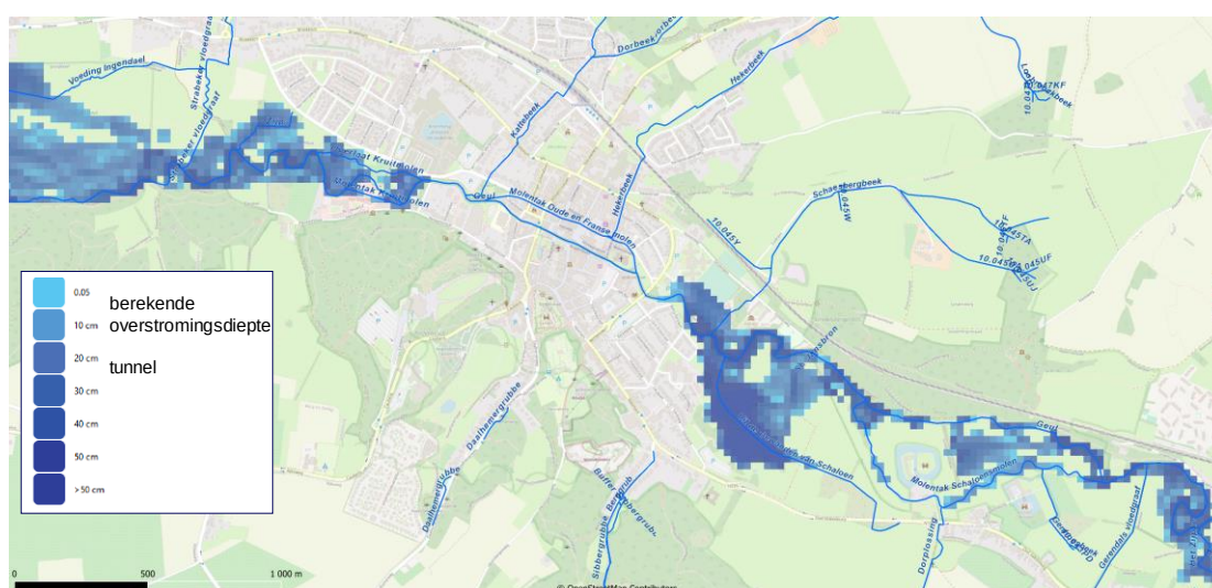
Figuur 26 Overstromingen rond Valkenburg na aanleg van twee tunnelbuizen met elk een diameter van 3.5 m
