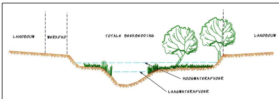
Figuur 28 Een voorbeeld van een accoladeprofiel, waarbij de lager gelegen zones langs de beek zijn ingericht als natuur (figuur overgenomen van https://lokaleregelgeving.overheid.nl/CVDR406842 )
