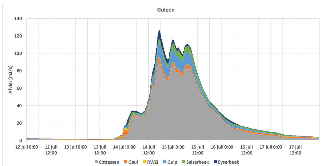
Figuur 16 Berekende afvoer net ten noorden van Gulpen, na samenkost van alle zijbeken. De herkomst van het water uit de verschillende deelstroomgebieden is met kleur aan gegeven
