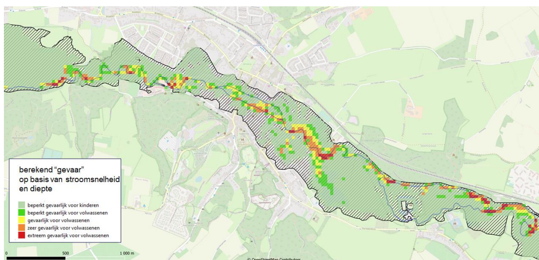
Figuur 23 Indicatie van gevaar (hazard) op basis van stroomsnelheid en diepte volgens methode AIDR 2017 (zie bijlage C)
