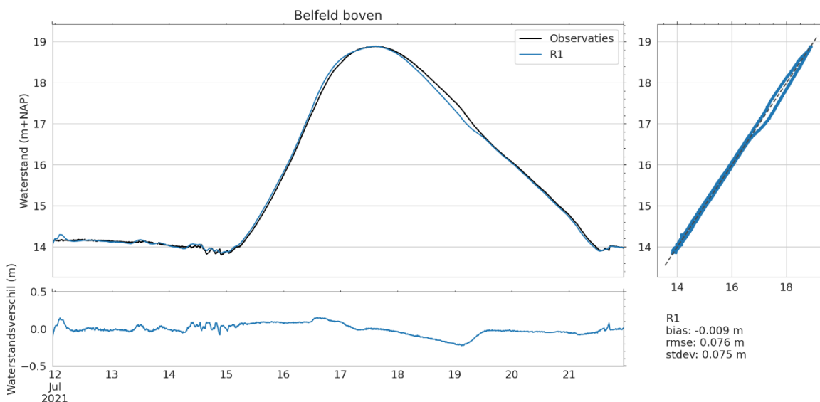
Figuur B-2: Validatie van Maasmodel 2D bij Belfeld
