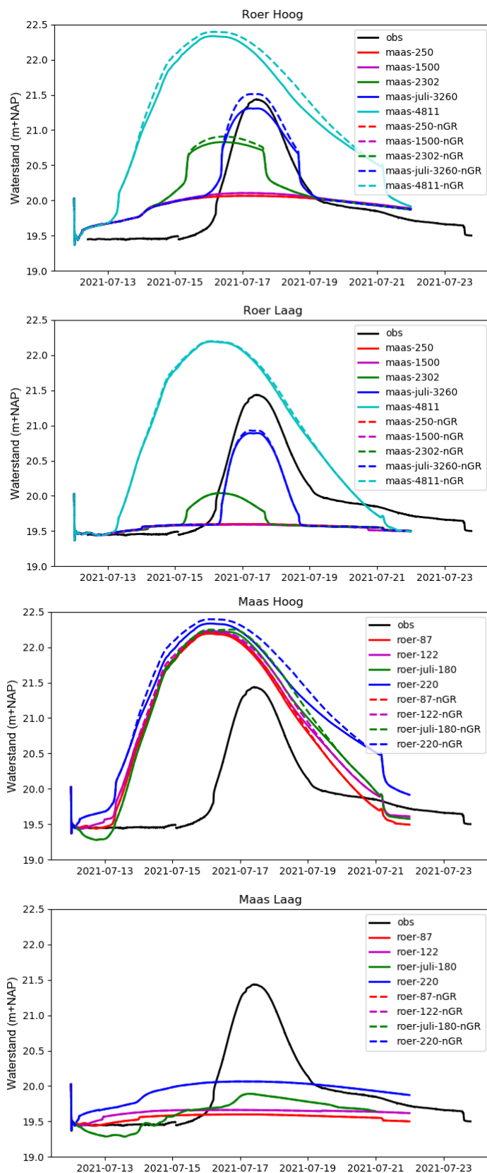
Figuur 3-8: Waterstanden bij meetpunt Roermond Andersonweg bij balgstuw Hoge Bat bij verschillende Maas- en Roerafvoeren. Roer hoog staat voor een afvoer van 220 m 3 /s. Bij Roer laag is een afvoer van 87 m 3 /s aangenomen. Maas hoog komt overeen met een Maasafvoer van 4811 m 3 /s en Maas laag met 250 m 3 /s. nGR geeft de scenario's zonder Roer-overlaat weer
