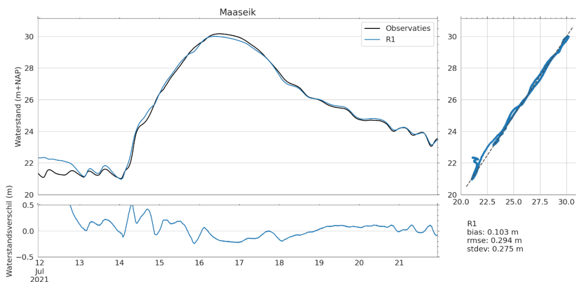
Figuur B-1: Validatie van Maasmodel 2D bij Maaseik
