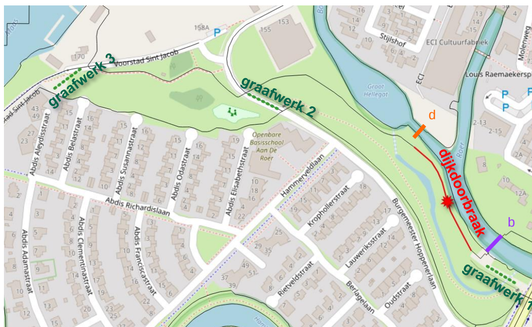
Figuur 2-3: Locatie van de gesimuleerde dijkdoorbraak (rode lijn) en locaties waar graafwerk uitgevoerd moet worden (groene stippellijnen) bij inzet van de Roer-overlaat. Verder illustreert b de zuidelijke keersluis en d de stuw Groot Hellegat
