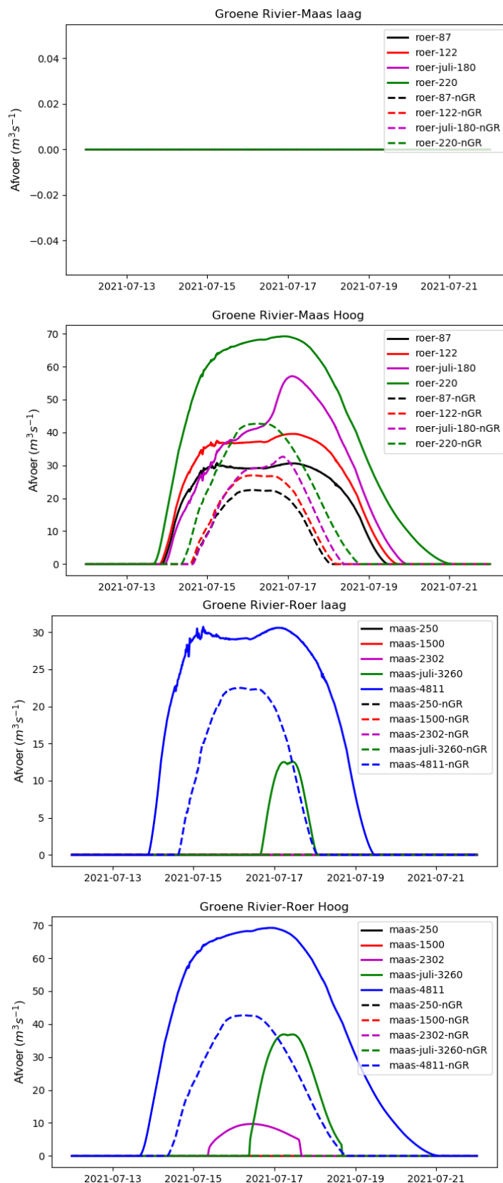
Figuur 3-9: Tijdsverloop van de afvoer door de Roer-overlaat met de meest extreme scenario's. Roer hoog staat voor een afvoer van 220 m³/s. Bij Roer laag is een afvoer van 87 m³/s aangenomen. Maas hoog komt overeen met een Maasafvoer van 4811 m³/s en Maas laag met 250 m³/s. nGR geeft de scenario's zonder Roer-overlaat weer
