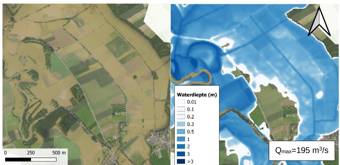
Figuur A-1: De verschillende afvoersimulaties voor de Roer bij Stah
