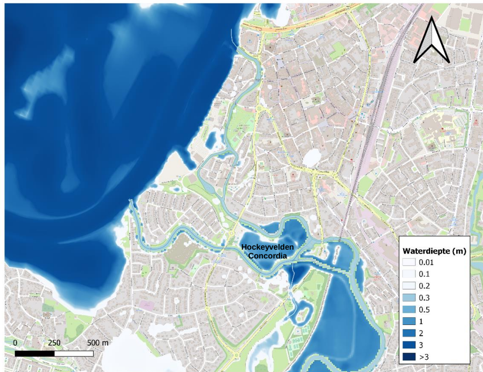
Figuur 3-1: Kaart met de gemodelleerde maximale overstroming van hoogwater juli 2021. De modelberekening geeft de maximale overstroming op 18 juli om 16:00 uur
