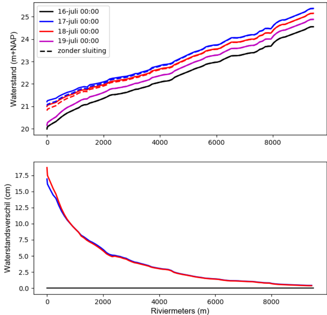
Figuur 3-11: Langsprofilen bovenstrooms van balgstuw Hoge Bat. De bovenste figuur toont de gemodelleerde waterstanden die zijn berekend met real-time control op de sluisdeuren (doorgetrokken lijn) en zonder real-time control, dus met open sluisdeuren (stippellijn). In het modelscenario met real-time control zijn de deuren gesloten op 16 juli om 6:00 uur en geopend op 18 juli om 20:00 uur. Er is dus enkel verschil in de modelsimulatie van het langsprofiel voor 17 juli om 0:00 uur en 18 juli om 0:00 uur. Dit verschil in berekende waterstand met gesloten en open sluisdeuren is getoond in de onderste figuur, waarbij de kleuren refereren aan de tijdstippen in de legenda. De referentie (km 0) ligt bij balgstuw Hoge Bat
