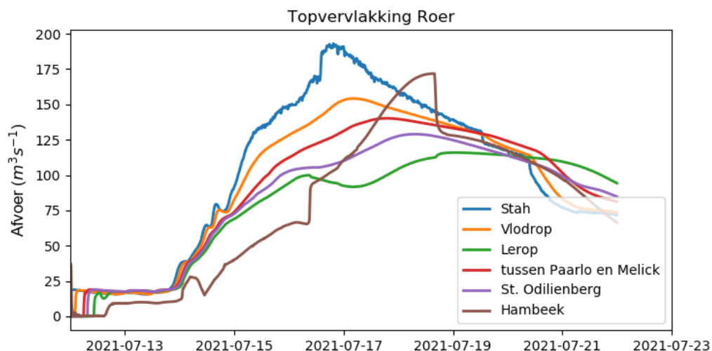
Figuur A-5: De gemodelleerde topvervlakking in de Roer met een maximale afvoergolf van 195 m³/s bij Stah. N.B. het vreemde afvoergolpatroon in de Hambeek wordt veroorzaakt door het samenvallen van de afvoergolf op de Maas
