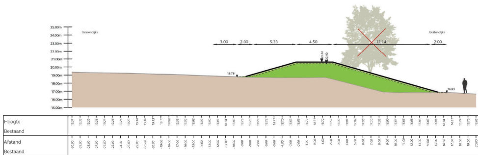
Dwarsprofiel dijkvak DV11-03 Schaal 1:200
