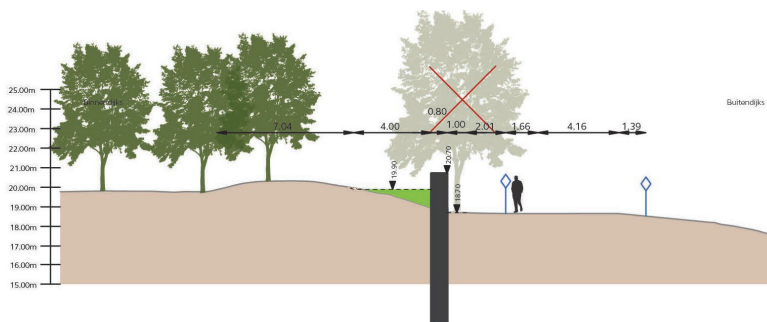
Dwarsprofiel dijkvak DV12-02
