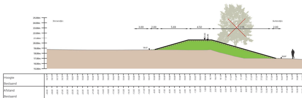
Dwarsprofiel dijkvak DV11-02 Schaal 1:200
