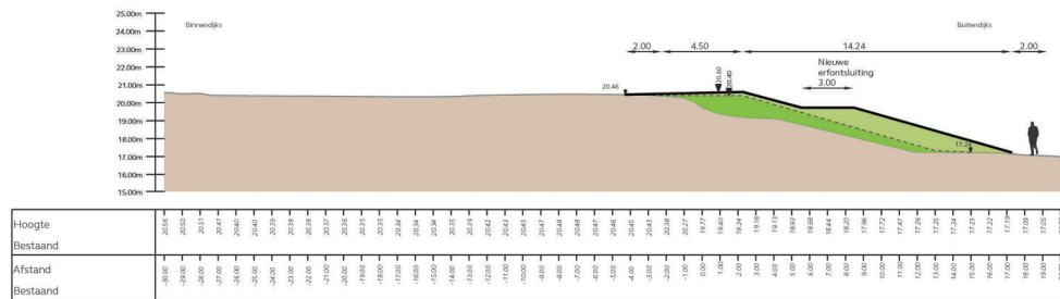
Dwarsprofiel dijkvak DV11-01 Schaal 1:200
