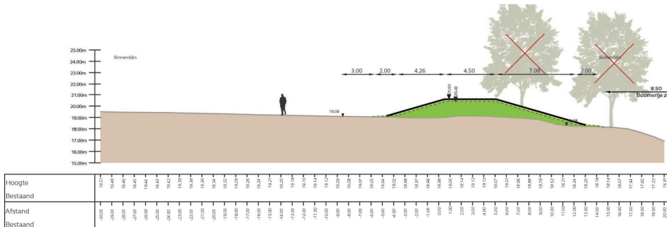
Dwarsprofiel dijkvak DV11-04 Schaal 1:200
