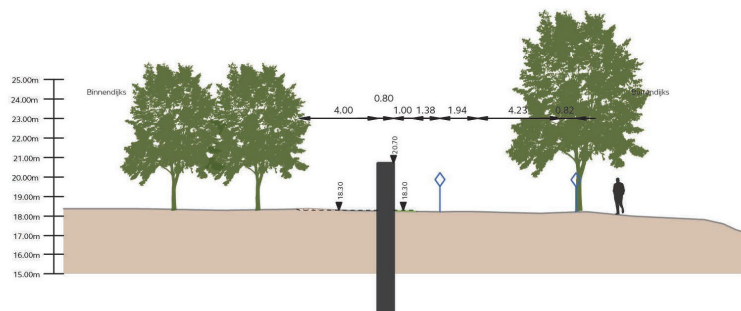
Dwarsprofiel dijkvak DV12-01
