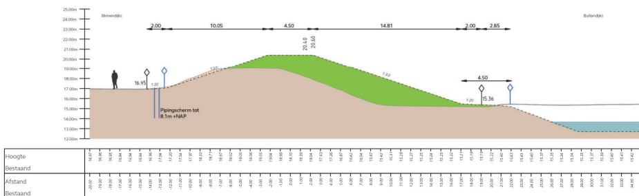
Dwarsprofiel dijkvak DV08-02 Schaal 1:200
