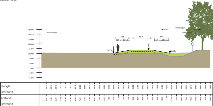
Dwarsprofiel dijkvak DV03-02 Schaal 1:200
