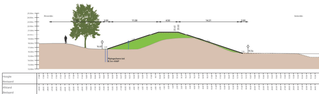
Dwarsprofiel dijkvak DV08-03 Schaal 1:200
