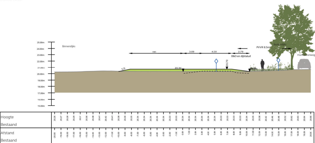
Dwarsprofiel dijkvak DV03-03 Schaal 1:200
