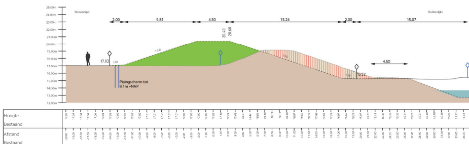
Dwarsprofiel dijkvak DV06-01 Schaal 1:200
