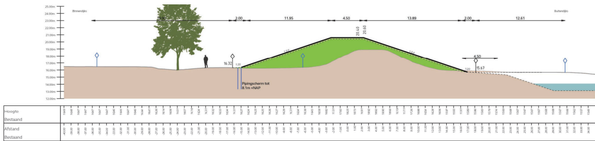
Dwarsprofiel dijkvak DV08-04 Schaal 1:200
