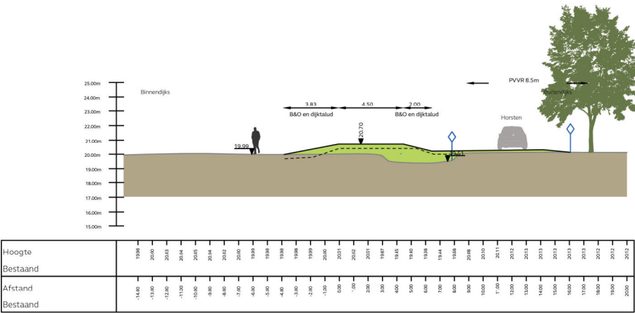
Dwarsprofiel dijkvak DV03-01 Schaal 1:200
