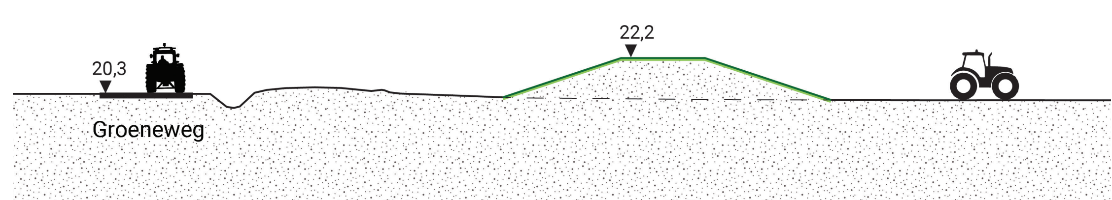
Dijkvak 3
