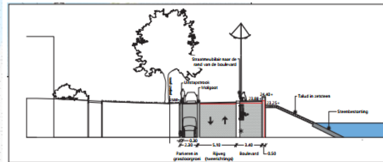
principedwarsdoorsnede Maasboulevard
