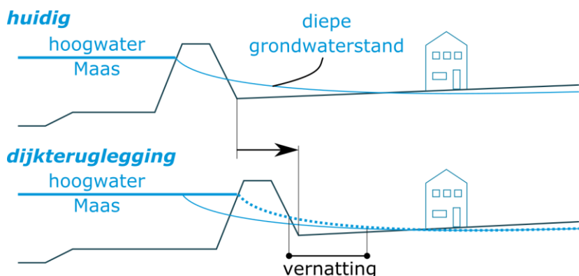
Afbeelding 13.2 Schematische doorsnede effect dijkeruglegging op grondwaterstand
