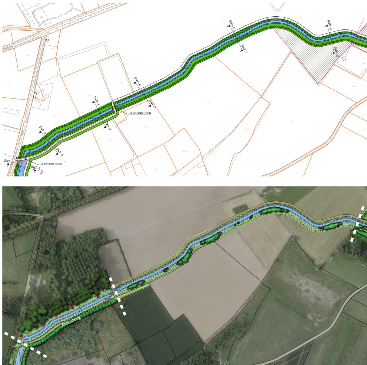
Figuur 5-13 Deeltraject B. Boven: inpassend ontwerp. Onder: Luchtfoto met landschappelijke inpassing.
