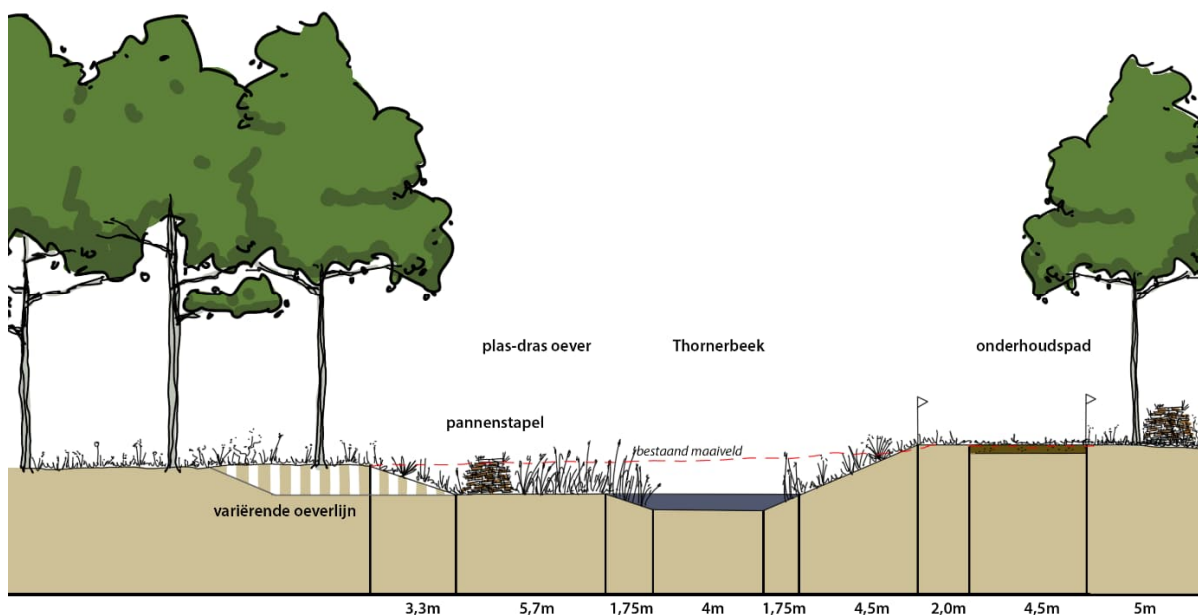
Figuur 5-15 Doorsnede t.h.v. Erkesteeg
