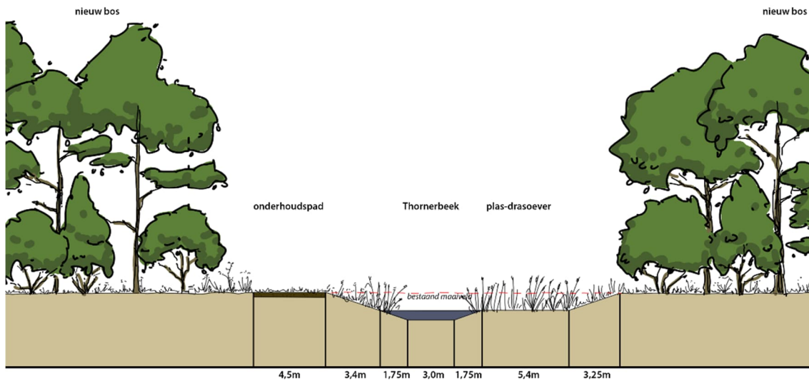
Figuur 5-19 Doorsnede t.h.v. Meggelveld
