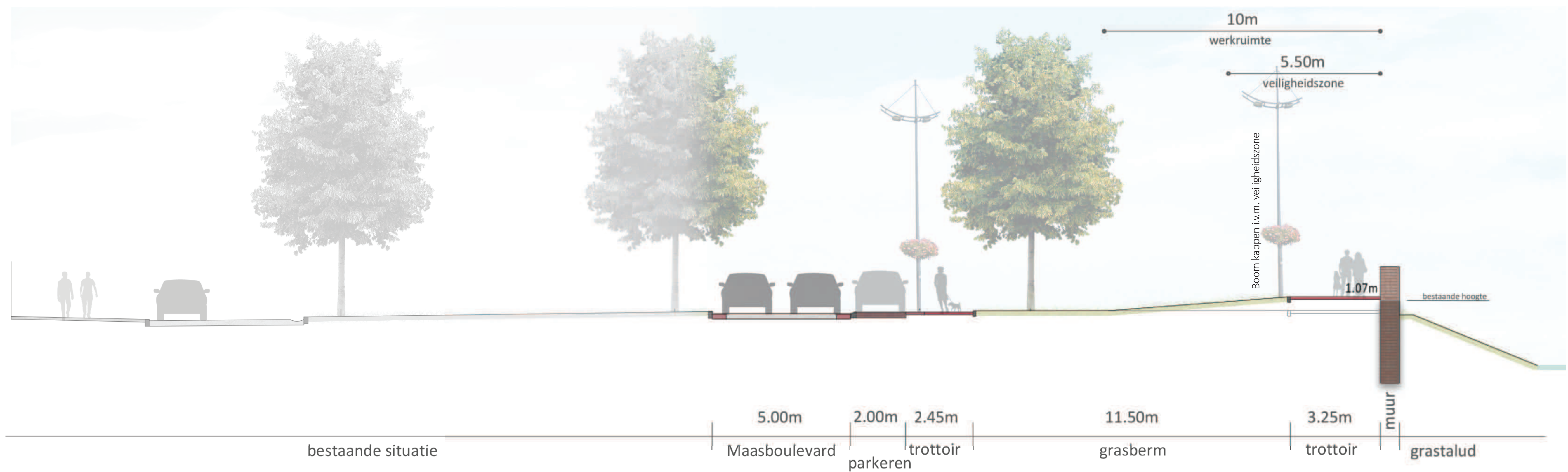
Doorsnede A: situatie zichtjaar 2125 hoogte muur: 107 cm
