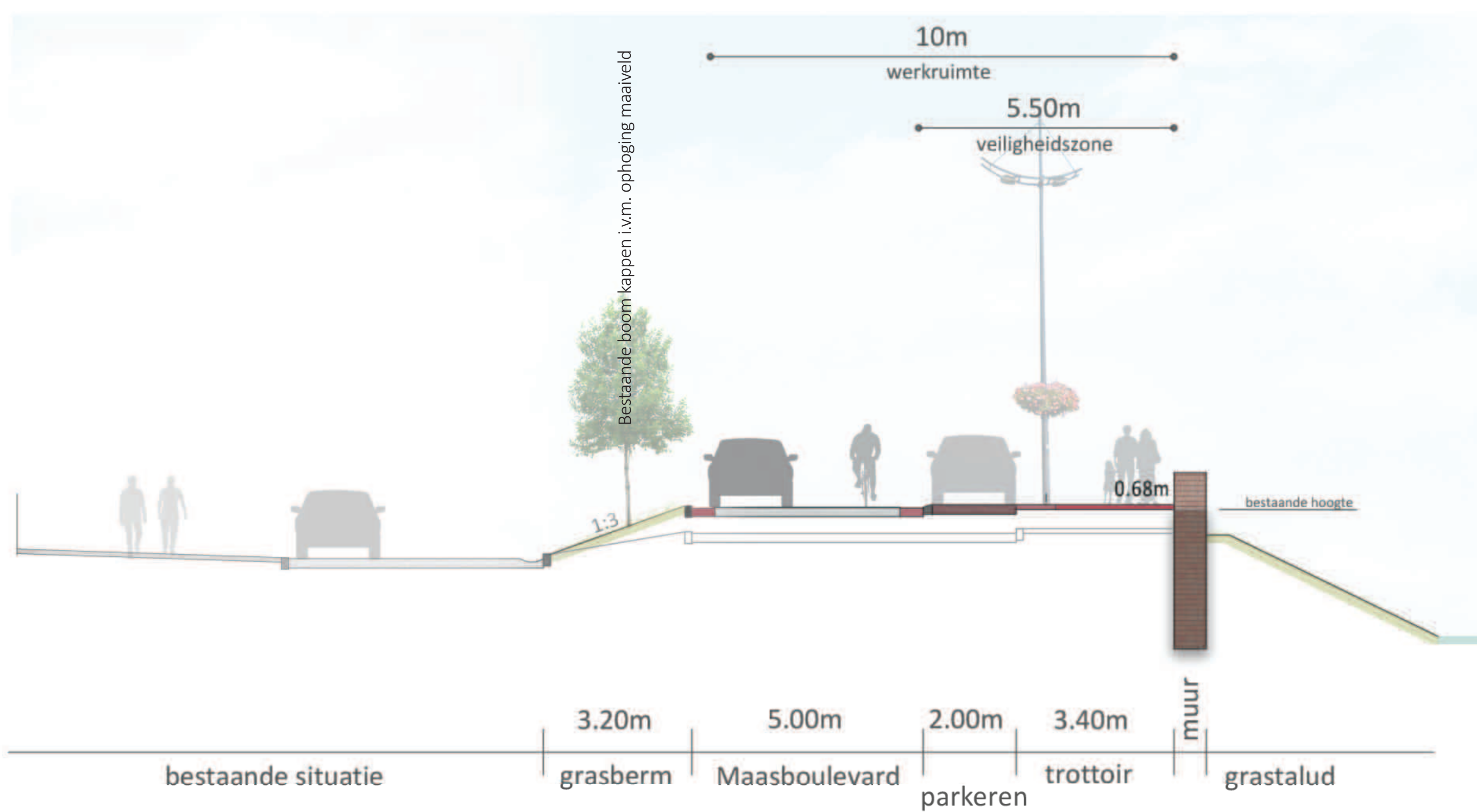
Doorsnede B: zichtjaar 2075 met opgehoogd maaiveld hoogte muur: 68 cm
