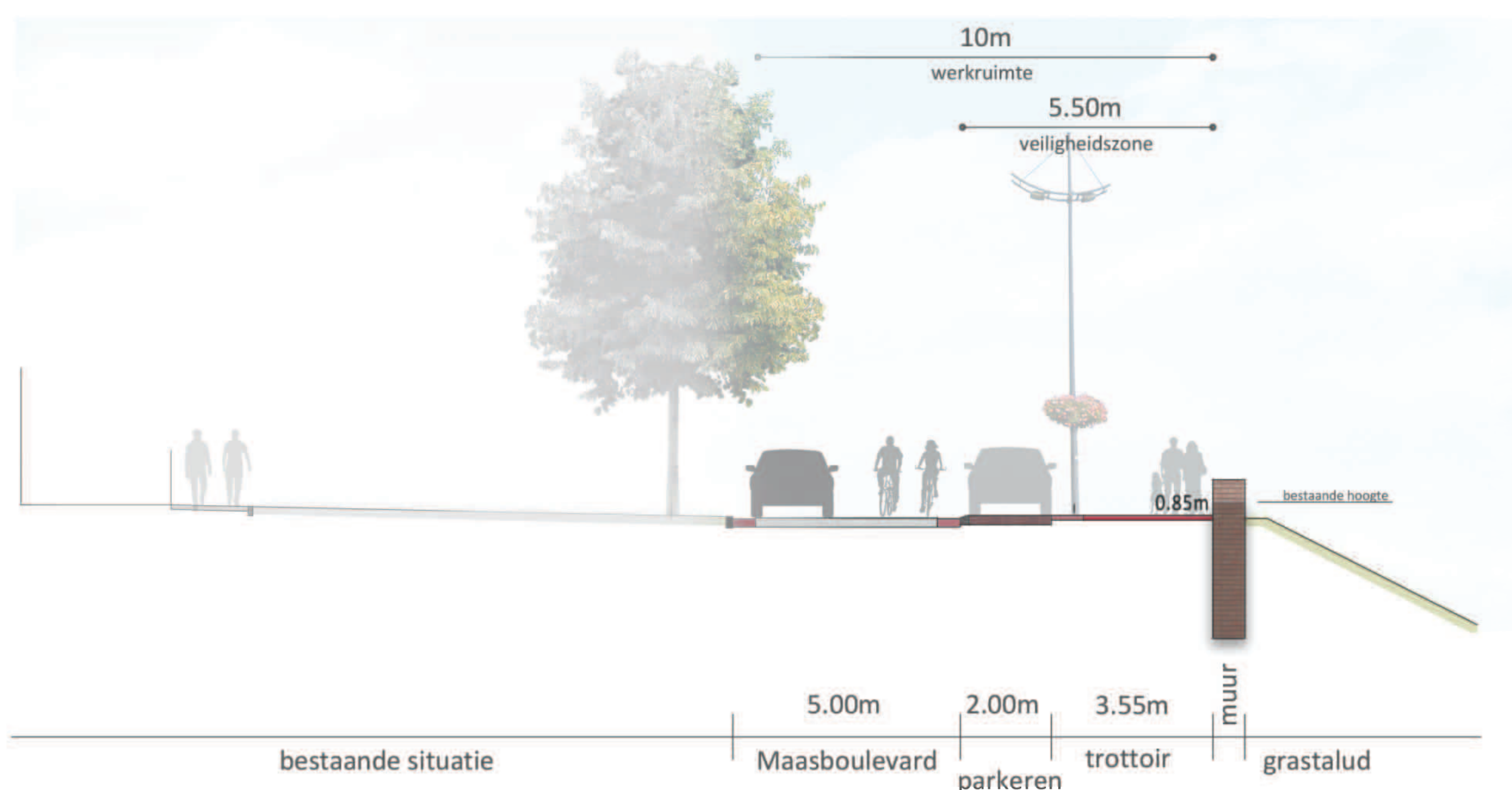
Doorsnede C: situatie tot 2075 hoogte muur: 85 cm
