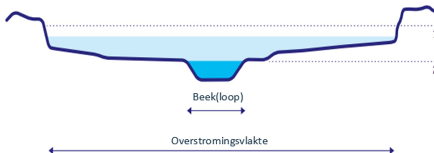
Figuur 5-2 Principeprofiel van een beek met R-type 5. (Handboek geomorfologisch beekherstel, Stowa).
