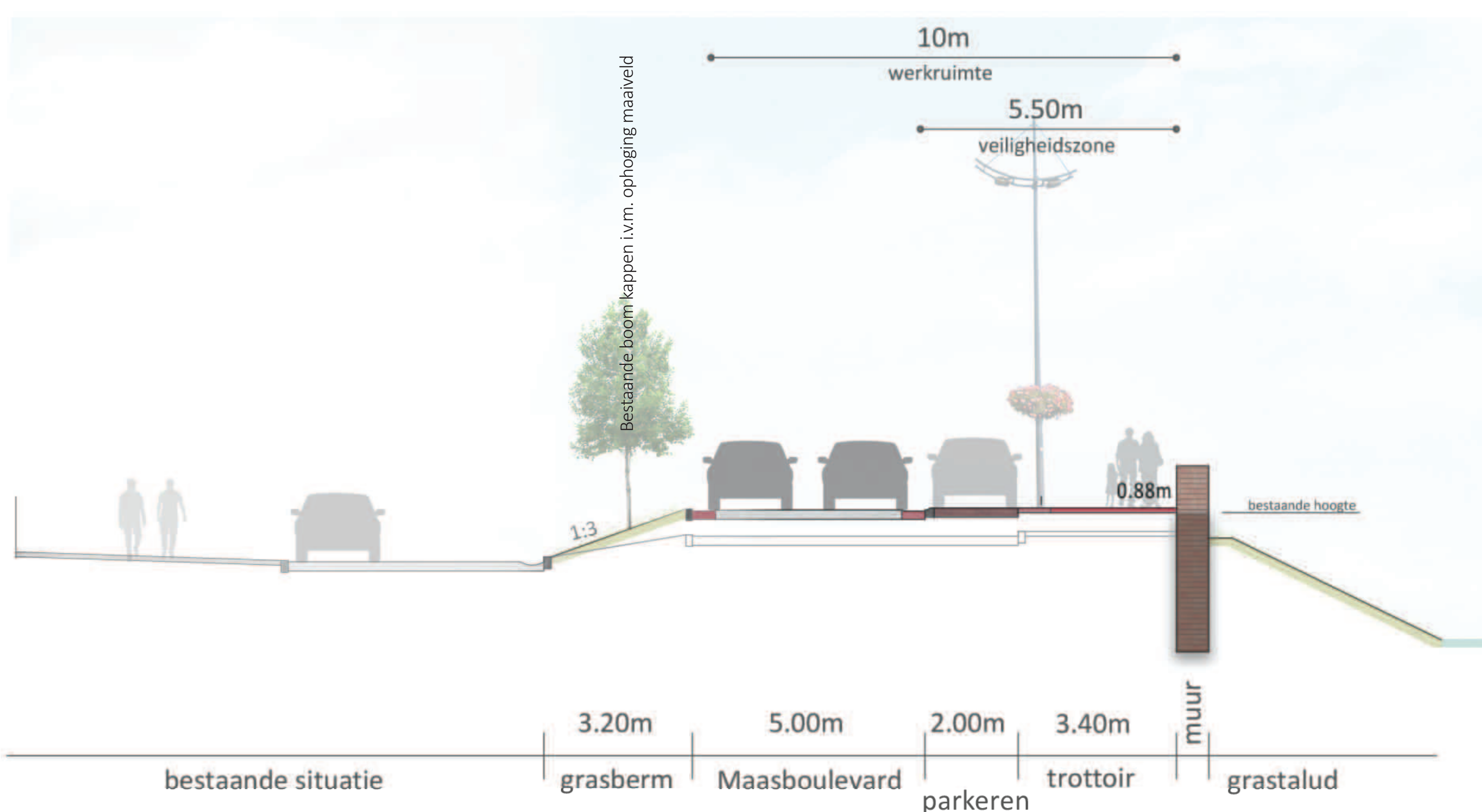
Doorsnede B: zichtjaar 2125 hoogte muur: 88 cm
