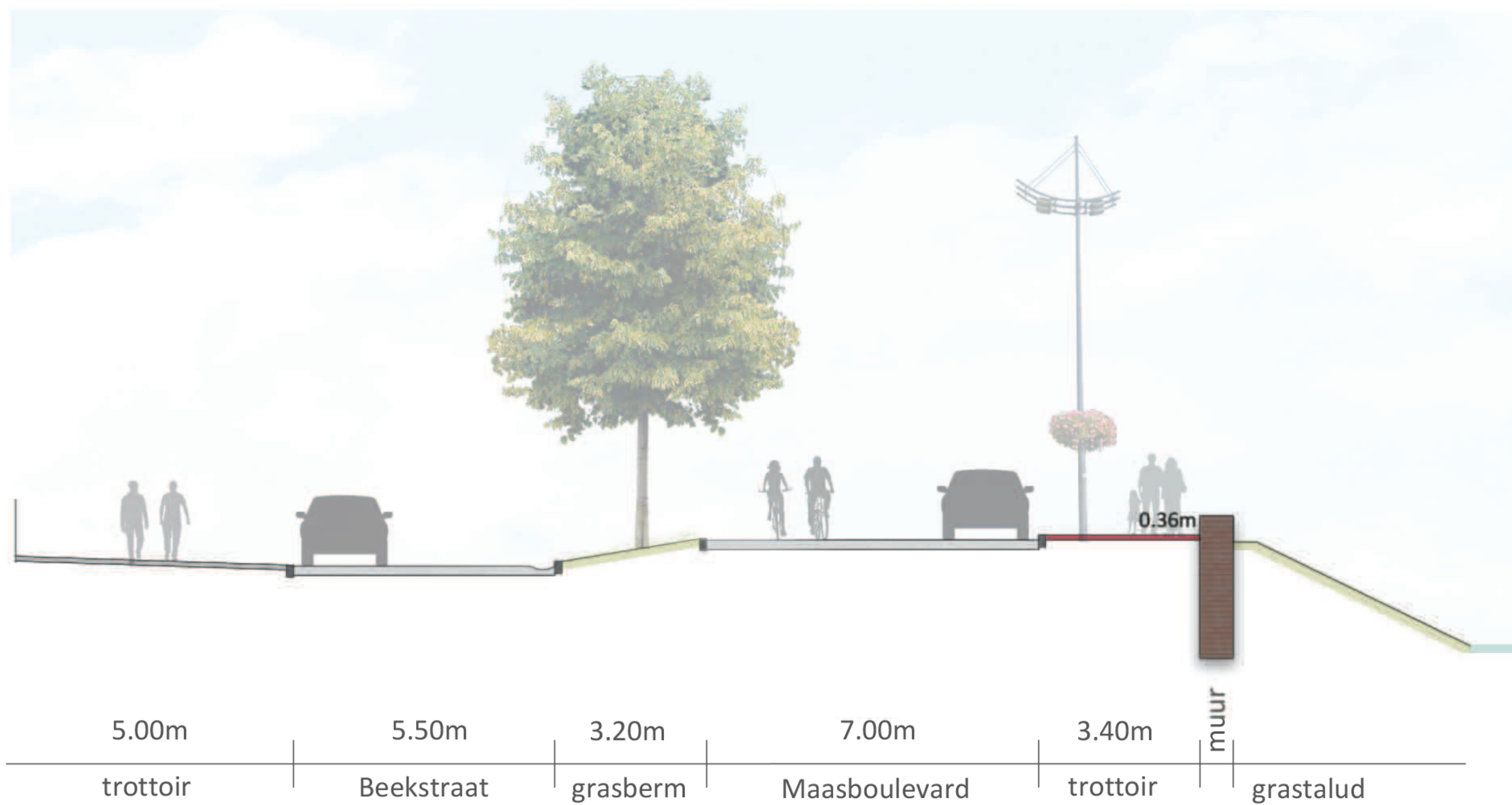
Doorsnede B: bestaande situatie hoogte muur: 36 cm
