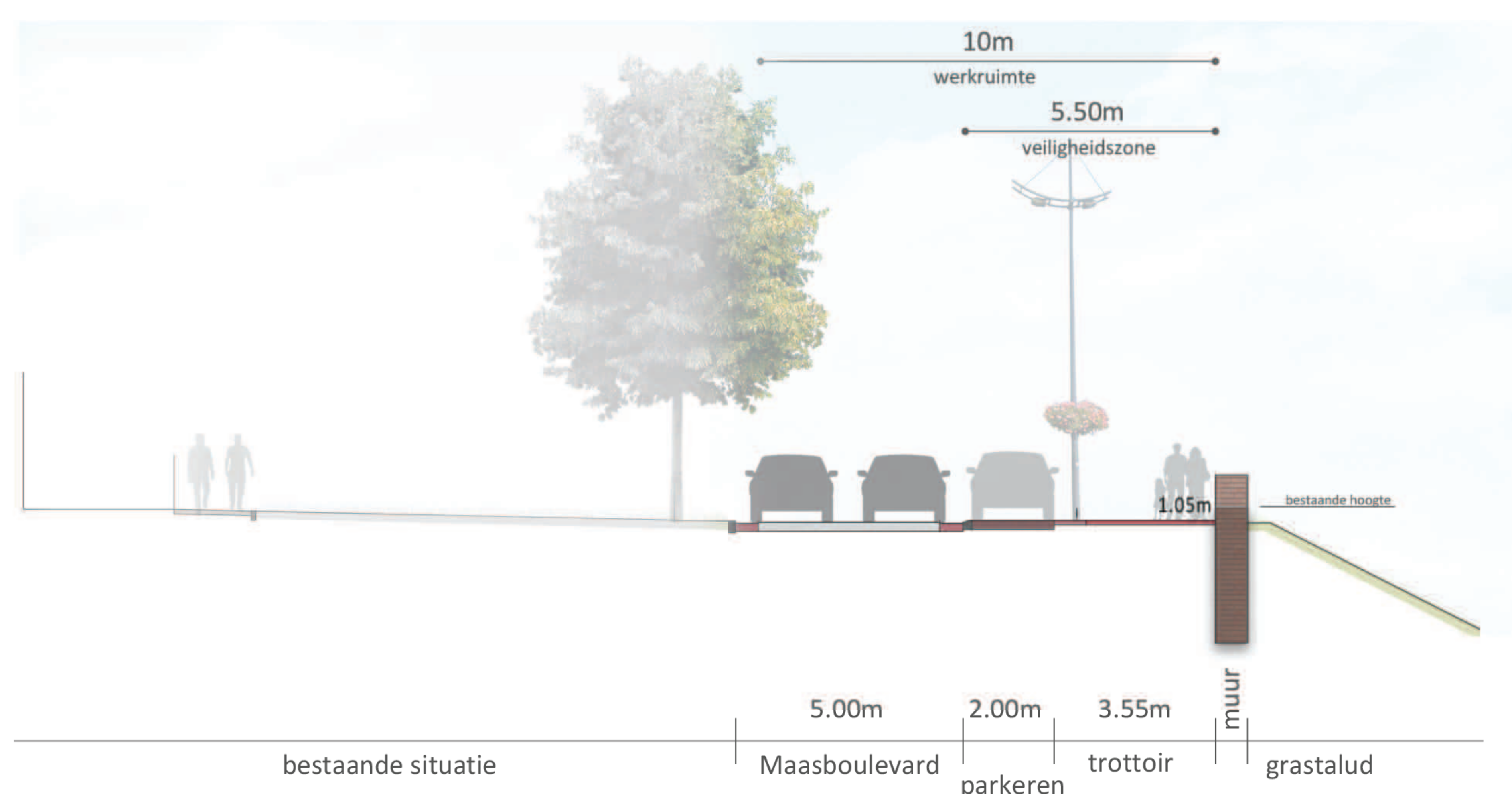
Doorsnede C: situatie vanaf 2075 tot 2125 hoogte muur: 105 cm
