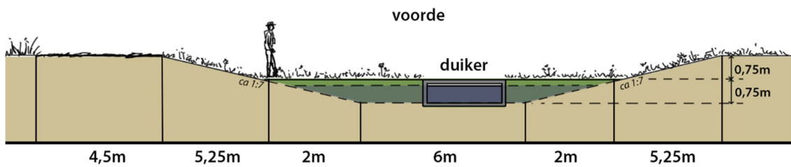
Figuur 5-10 Principedoorrsnede doorwaadbare plaats: voorde met duiker
