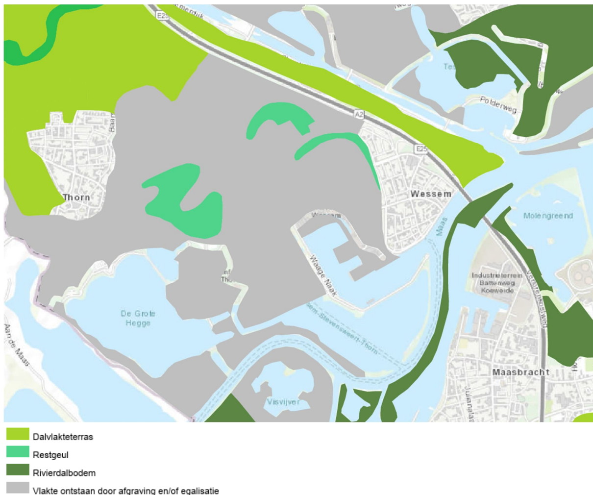
Figuur 2-1 Geomorfologische kaart
