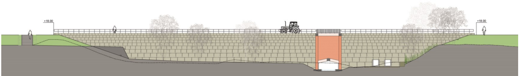
Aanzicht van de kistdam vanaf buitendijks (zicht vanaf natuurgebied Barbara's Weerd)
