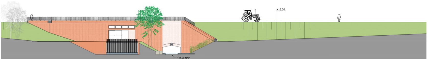
Aanzicht van de kistdam vanaf binnendijks (zicht vanaf de Wijmarsche Watermolen)
