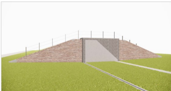
Aansluiting op dijk
