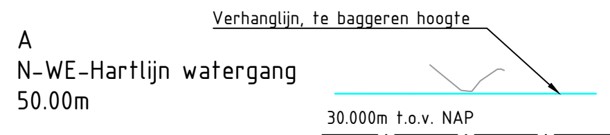
Lengteprofiel Watergang Schaal 1:500 1:50
