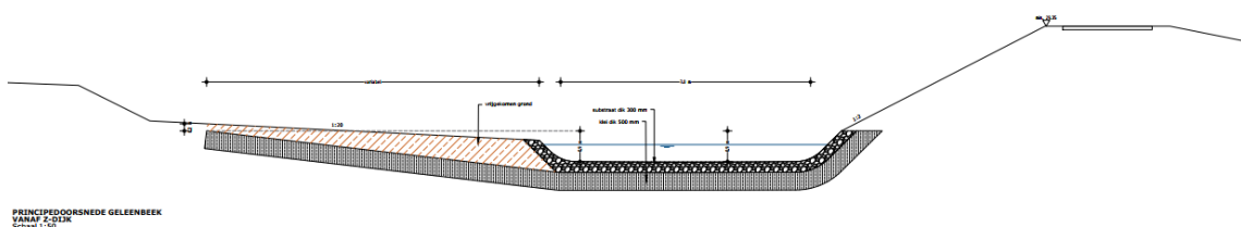
Afbeelding 1. Principe profiel Geleenbeek met bodemafdichting
