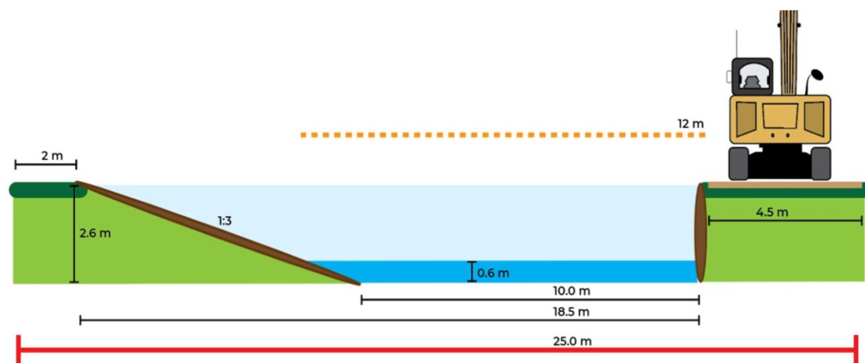
Figuur 3-27 Principe profiel deeltraject A, inpassing terrein voormalige dakpannenfabriek (hoogten op principe profiel zijn t.o.v. maaiveld en betreft de hoogte na inklinking)
