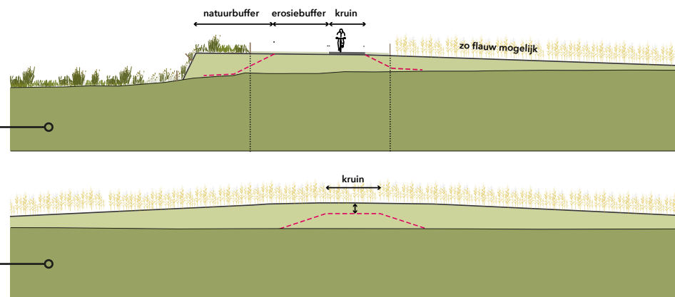
Figuur 5 - Twee innovatieve dijkconcepten in Limburg, de steilranddijk (boven) en de hoge gronddijk (beneden).
